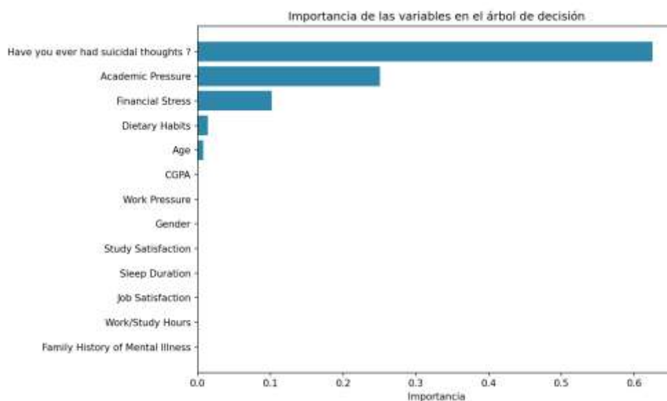
Figura 3. Importancia relativa de las variables en el árbol de decisión.
