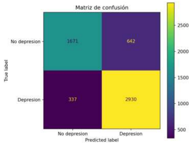
Figura 2. Matriz de confusión del árbol de decisión sobre el conjunto de prueba.
